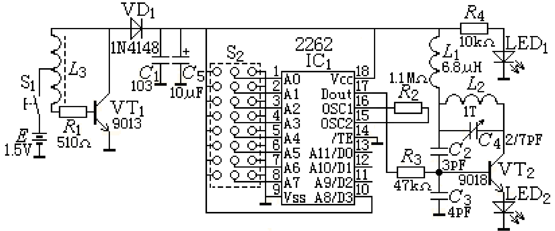
附图 3 控制电路图
